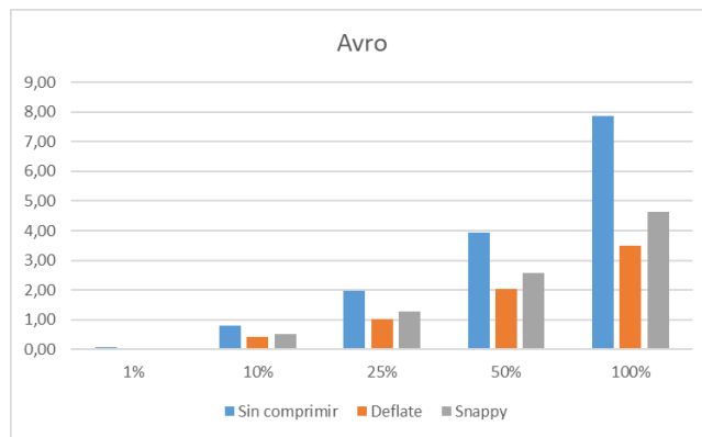
Figure 2: Comparación tabulada de memoria utilizada en la conversión a formato AVRO.
